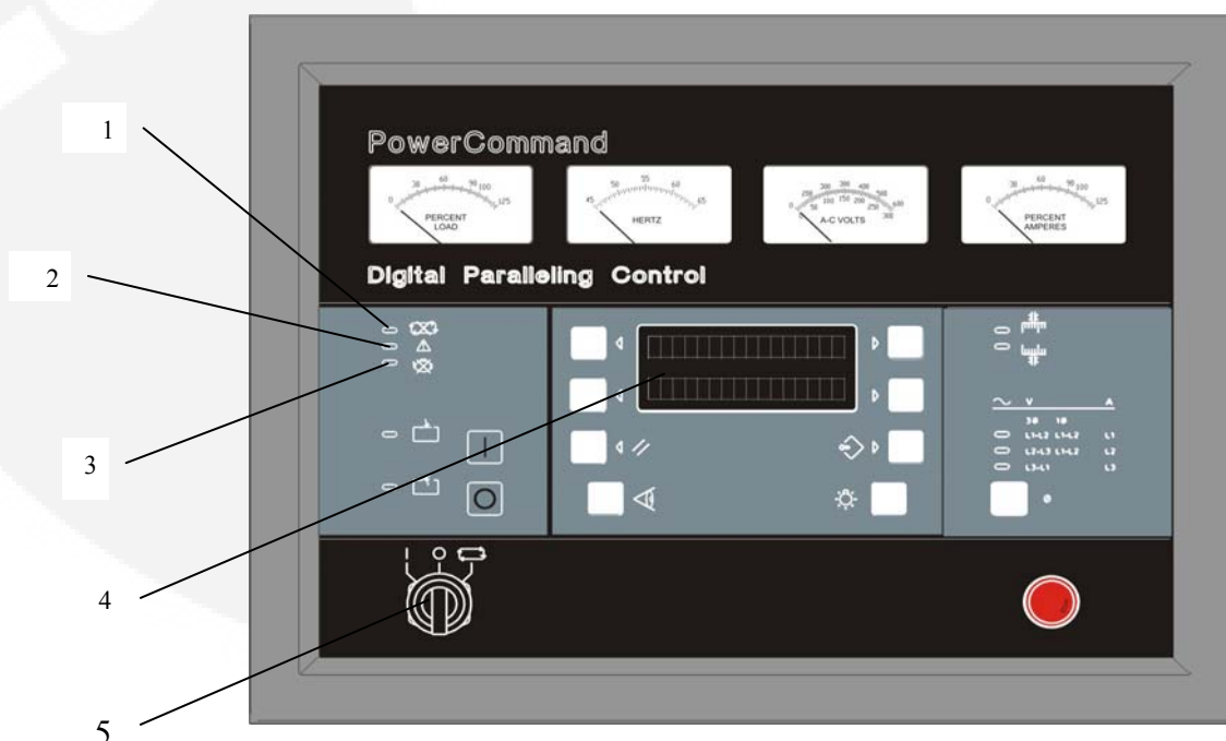
Рисунок 7-1 Лицевая панель
